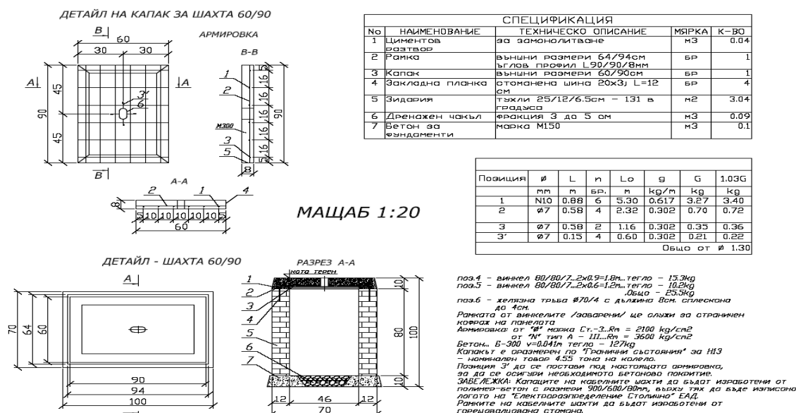
Фиг. 1. Кабелна шахта – единич
